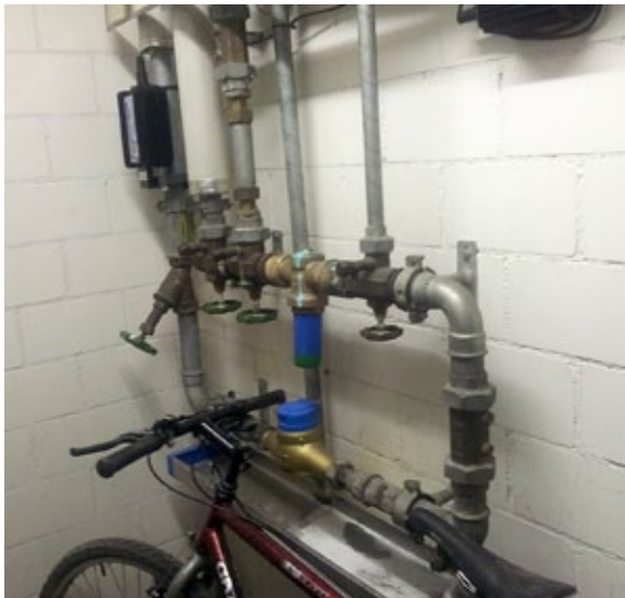
Distribution d'eau galvanisé, env. 1980 avec traitement d'eau « magnétique »
