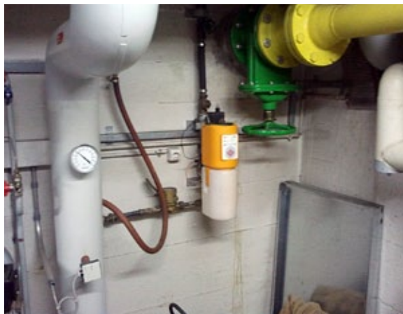
Impfchleuse «Impfbiene» für Phosphat, seit 1978 nicht mehr zugelassen
